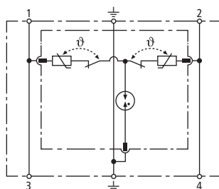
Prinzipschaltbild DR M 2P 255
