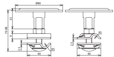
Maßbild FP D80 ET70 8.10 V2A
