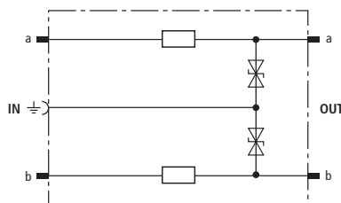
Prinzipschaltbild DRL RE 180
