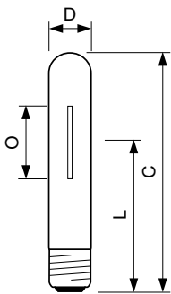
SON-T APIA Plus Xtra 50W E27
