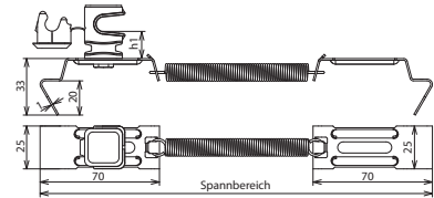
Maßbild DLH SS 8 H36 FG180.280 GR V2A
