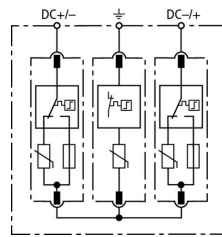
Prinzipialschaltbild DG M YPV SCI 1200
