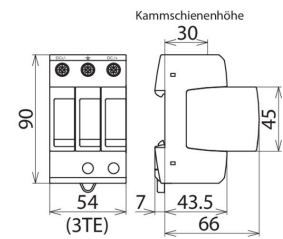
Maßbild DG M YPV SCI 1200
