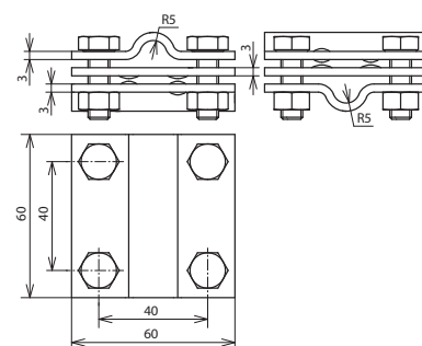
Maßbild KS 8.10 8.10 FL30 ZP STTZN
