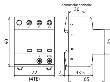
Maßbild DSH TNC 255
