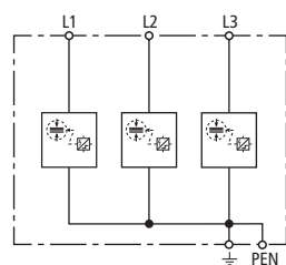
Prinzipschaltbild DSH TNC 255
