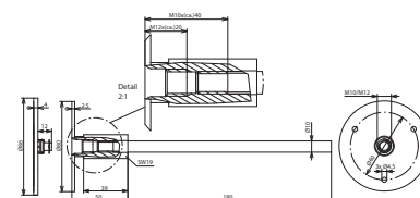
Maßbild EFPM M10 12 V4A L230 STTZN
