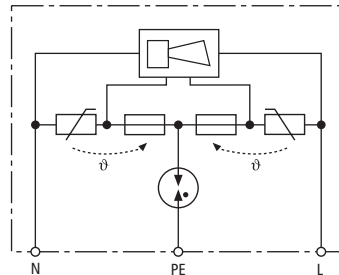
Prinzipschaltbild
