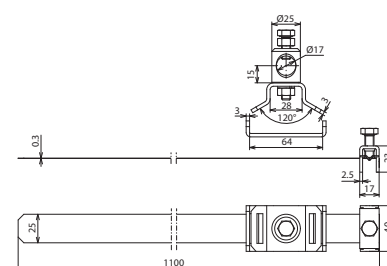
Maßbild BRS 50.300 BB16 8 V2A
