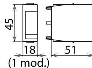
Maßbild DG PLU 180
