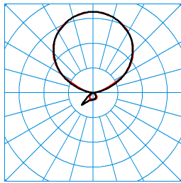
LuceoS S-U SMC PAW-IL 300-840 ETDI 05 (LEO1) TX369323 ■ C0 - C180 ■ C90 - C270 DIN 5040: E03 UTE: 0,08 D + 0,91 T CEN Flux Code: 53 86 96 8 100 49 82 98 92
