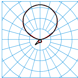
LuceoS S-U SMC PAW-IL 300-840 ETDI 05 (LEO2) TX369871 ■ C0 - C180 ■ C90 - C270 DIN 5040: E03 UTE: 0,08 D + 0,91 T CEN Flux Code: 53 86 96 8 100 49 82 98 92
