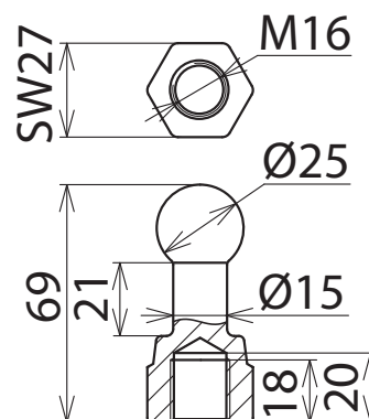
Maßbild KFP 25 M16
