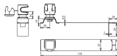
Maßbild DLH FS 8 H36 L170 GR V2A
