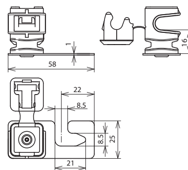
Maßbild DLH DS 8 H16 WPRO5 8 GR V2A
