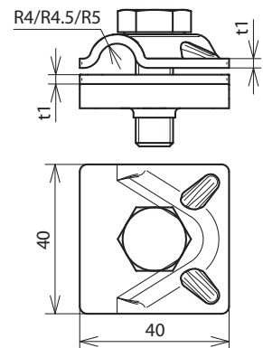
Maßbild MVK 8.10 SKM10X30 V2A
