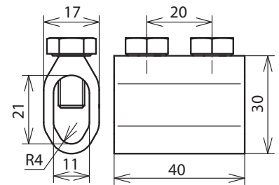
Maßbild TM 8.10 8 AL
