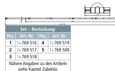
Maßbild EST SQL RW 4855 TA
