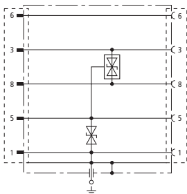
Prinzipschaltbild FS 9E PB 6
