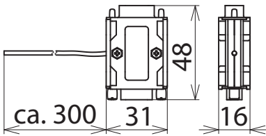
Maßbild FS 9E PB 6
