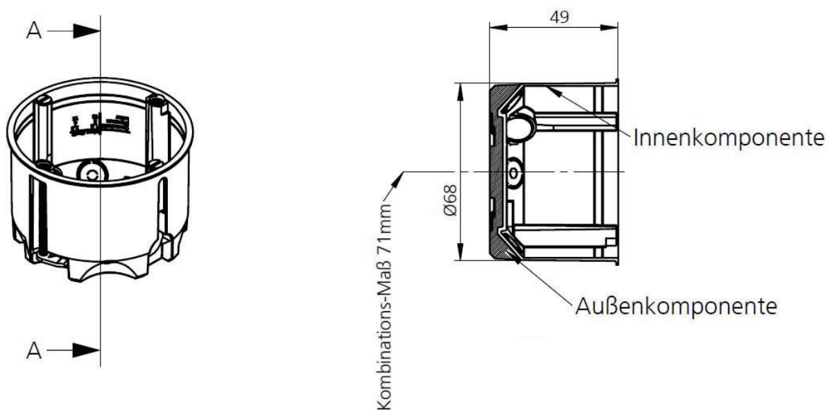
SCHNITT A-A
