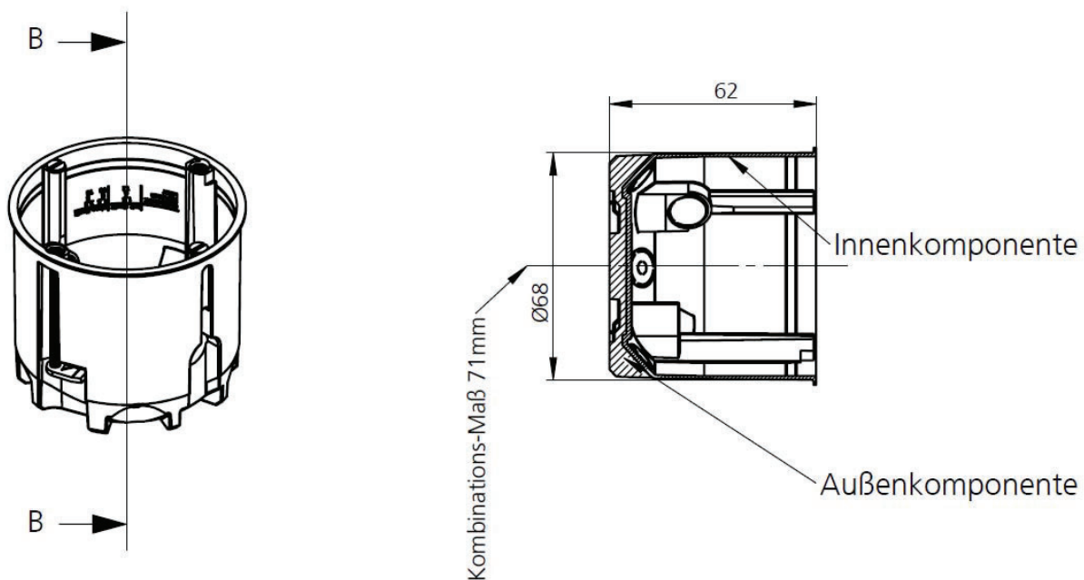
SCHNITT B-B
