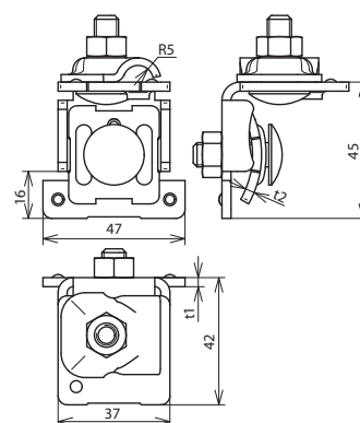
Maßbild FK KB 6.10 KBF0.7 8 W STTZN
