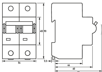
Maßzeichnung Gruppenansicht
