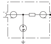
Prinzipschaltbild
