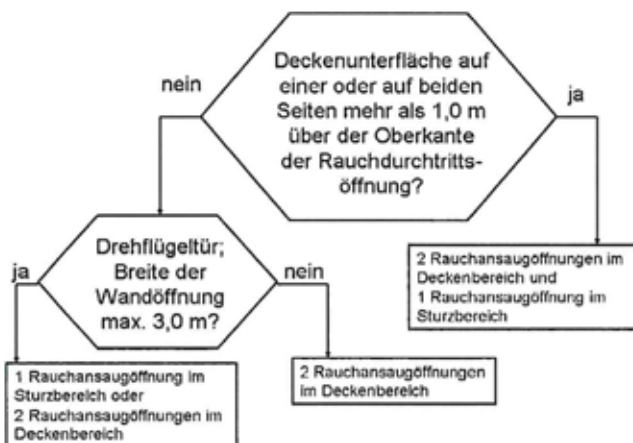
Bild 6: Entscheidungsdiagramm
