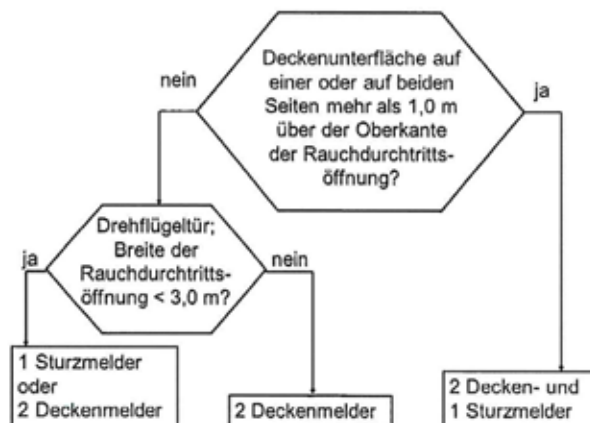
Bild 3: Entscheidungsdiagramm
