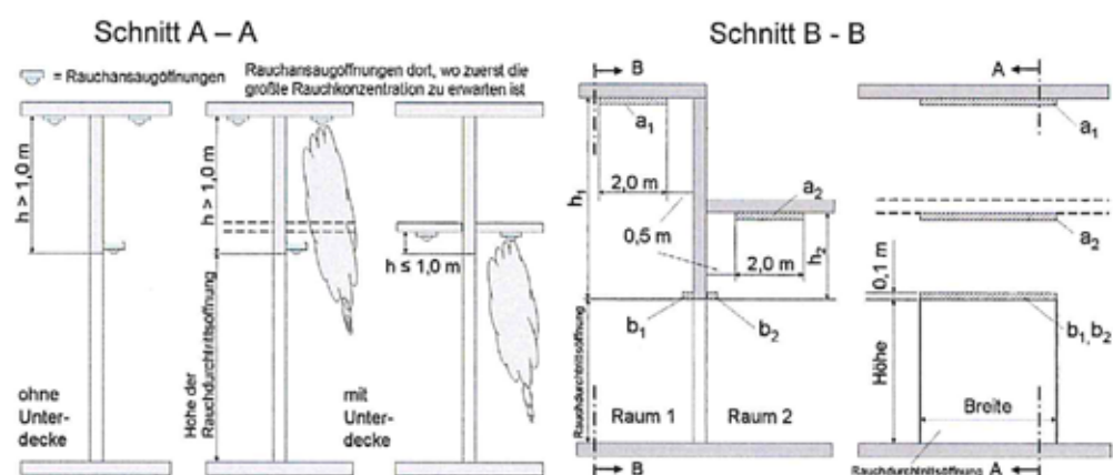
Bild 4: Maßgebende Höhe der Deckenunterfläche
