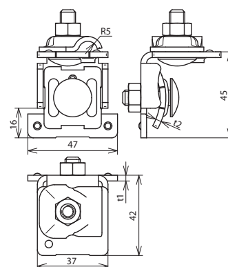
Maßbild FK KB 6.10 KBF0.7 8 W V2A
