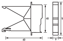
Maßzeichnung Gruppenansicht
