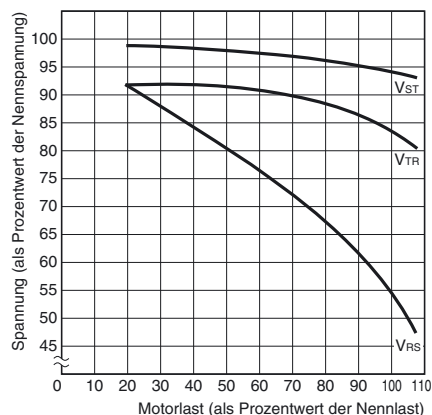
Kennliniendiagramm
