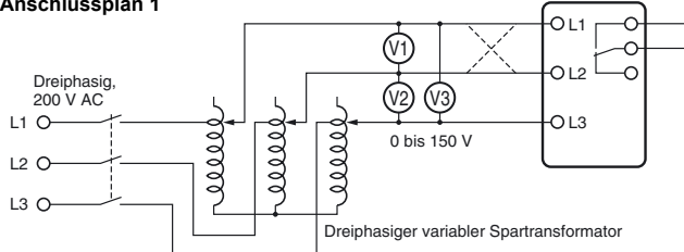
Anschlussplan 1
