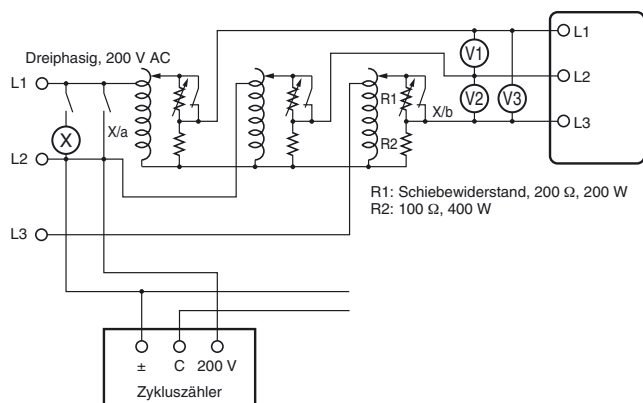
Anschlussplan 2
