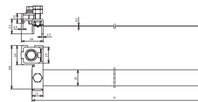
Maßbild BRS 27.89 AK1X10 2X6.8 GSG V2A
