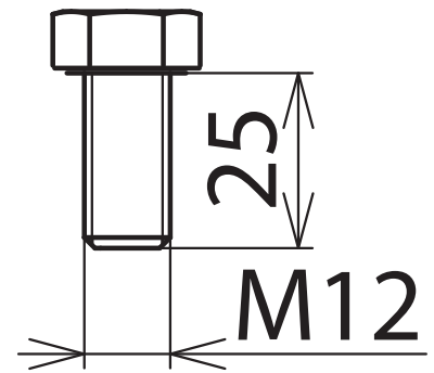
Maßbild SKS M12X25 V2A
