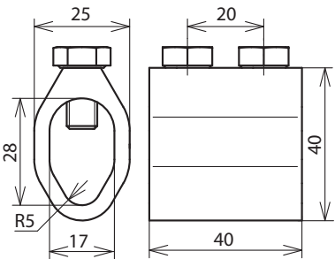
Maßbild TM 7.10 16 AL
