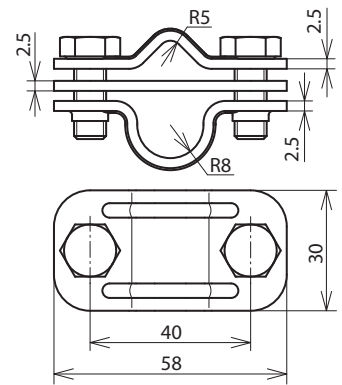
Maßbild UTK 8.10 16 ZP V2A
