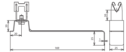
Maßbild DLH DG 8 H20 L169 WS V2A
