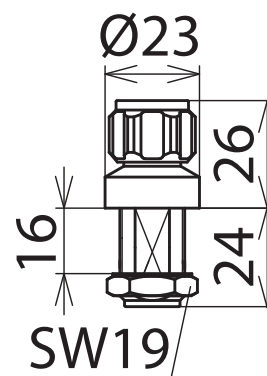
Maßbild DGA G N
