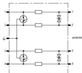
Prinzipialschaltbild BSP M4 BD 48
