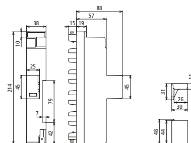
Maßbild DSH ZP B2 TT 255
