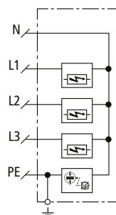
Prinzipschaltbild DSH ZP B2 TT 255
