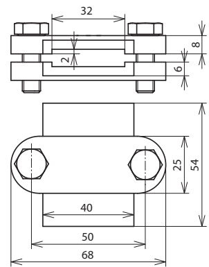
Maßbild VTK FL30 TGTZN
