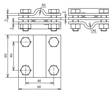
Maßbild KS 8.10 8.10 FL30 ZP V4A
