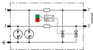
Prinzipschaltbild BCO ML2 BE 180
