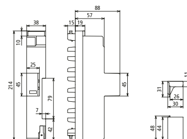
Maßbild DSH ZP 2 TNS 255
