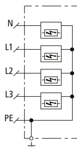
Prinzipschaltbild DSH ZP 2 TNS 255
