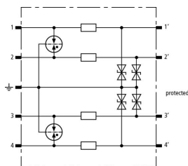
Prinzipialschaltbild BSP M4 BE 48
