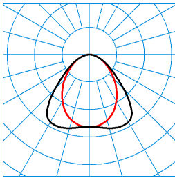
Cflex H1-E B 5500-840 EB3 01 TX039724
