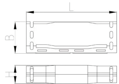
Maßbild VM EASY 5 TE M16
