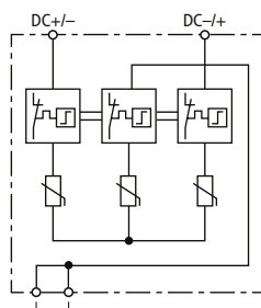
Prinzipschaltbild DCB YPV 1200
