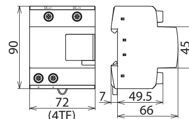
Maßbild DCB YPV 1200
