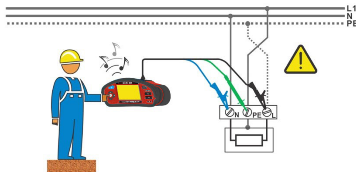
Abbildung 1.2: Vertauschte Leiter L und PE (Verwendung der 3-Leiter Prüflleitung)
