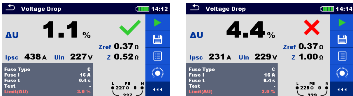
Abbildung 7.42: Beispiele für Ergebnisse der Spannungsfallmessung (Schritt 2)
