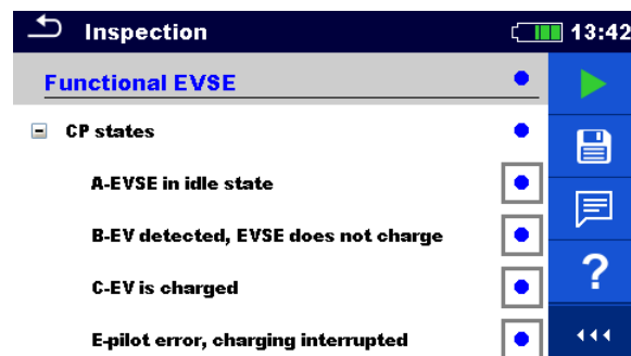
Abbildung 7.86: Beispiel für ein Ergebnis der Funktionsprüfung
