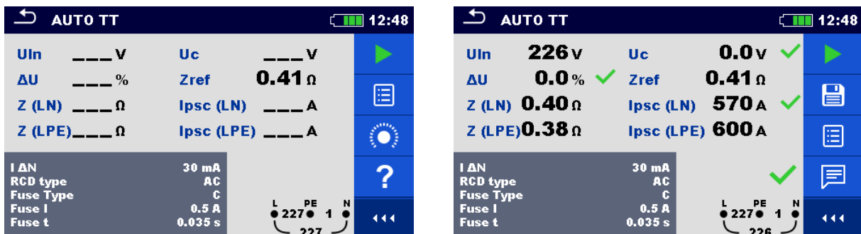
Abbildung 7.74: Beispiele für Ergebnisse der AUTO TT-Messung
