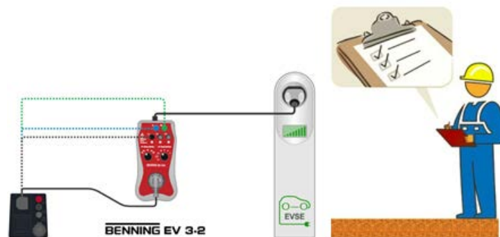
Abbildung 7.85: Funktionsprüfung
