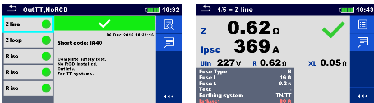
Abbildung 8.8: Ergebnisanzeige einer Einzelprüfung der Auto Sequence®
