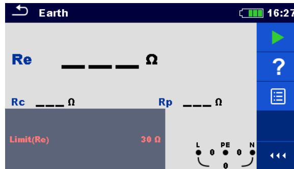
Abbildung 7.46 Menü Erde 3-Leiter
