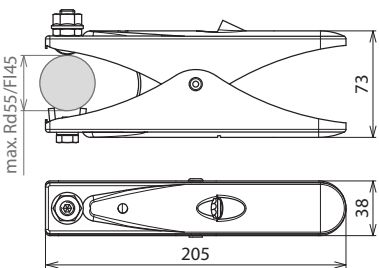
Maßbild EZ 55 FL45 ASM10 V2A
