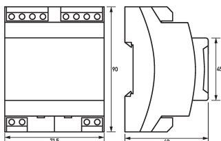
Maßzeichnung Gruppenansicht
