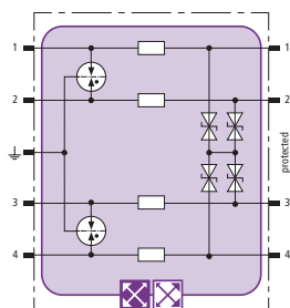
Prinzipschaltbild BXT ML4 BC 24
