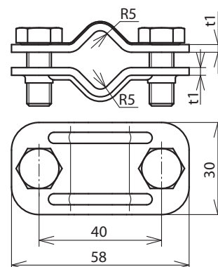
Maßbild UTK 8.10 8.10 STTZN
