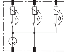
Prinzipschaltbild
